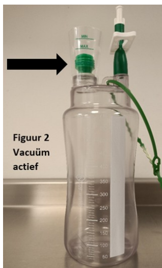
Figuur 2: Drainpot. Een actief vacuüm (links) en een verbroken vacuüm (rechts).
